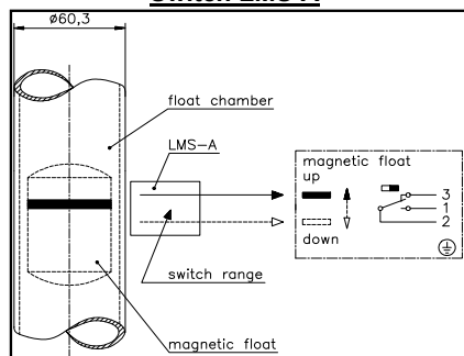
Switch LMS-A
